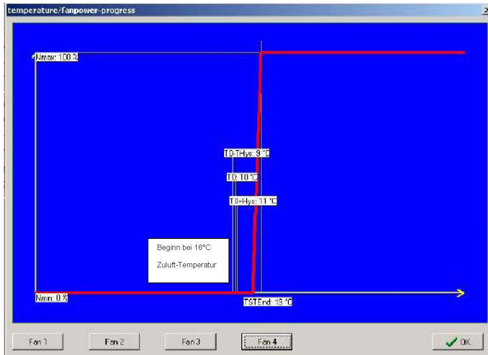
Kennlinie der Regelung des Dreivegventils (Werkseinstellung)
